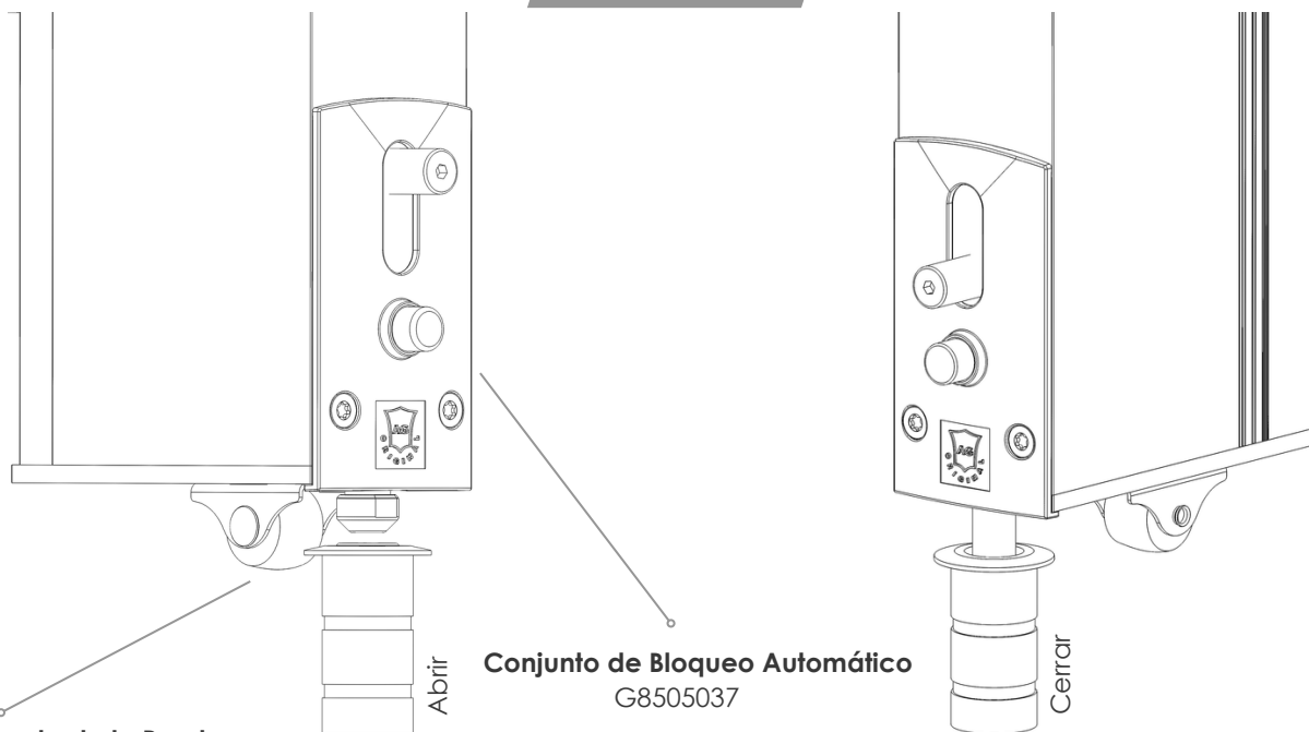
Airflex Rueda de la Puerta G8505035
