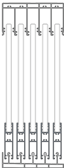
SliderNext con umbral de carril inferior
