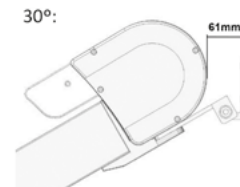
Medidas principales montaje PRO AIR.
